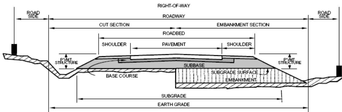
Roadway Nomenclature
